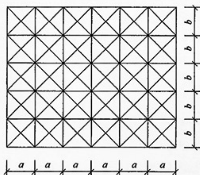
图 17 矩形风管测点布置图
