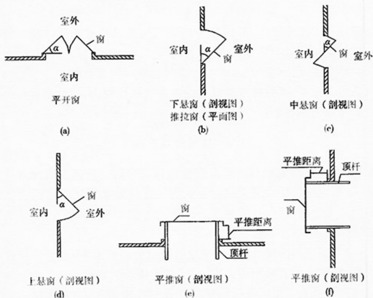
图 6 可开启外窗的示意图
