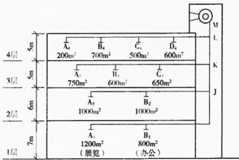
图 8 排烟系统示意图
