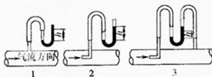
图 19 用 U 形管压力计测定风压
