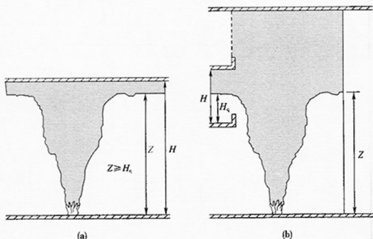
图9 最小清晰高度示意图
