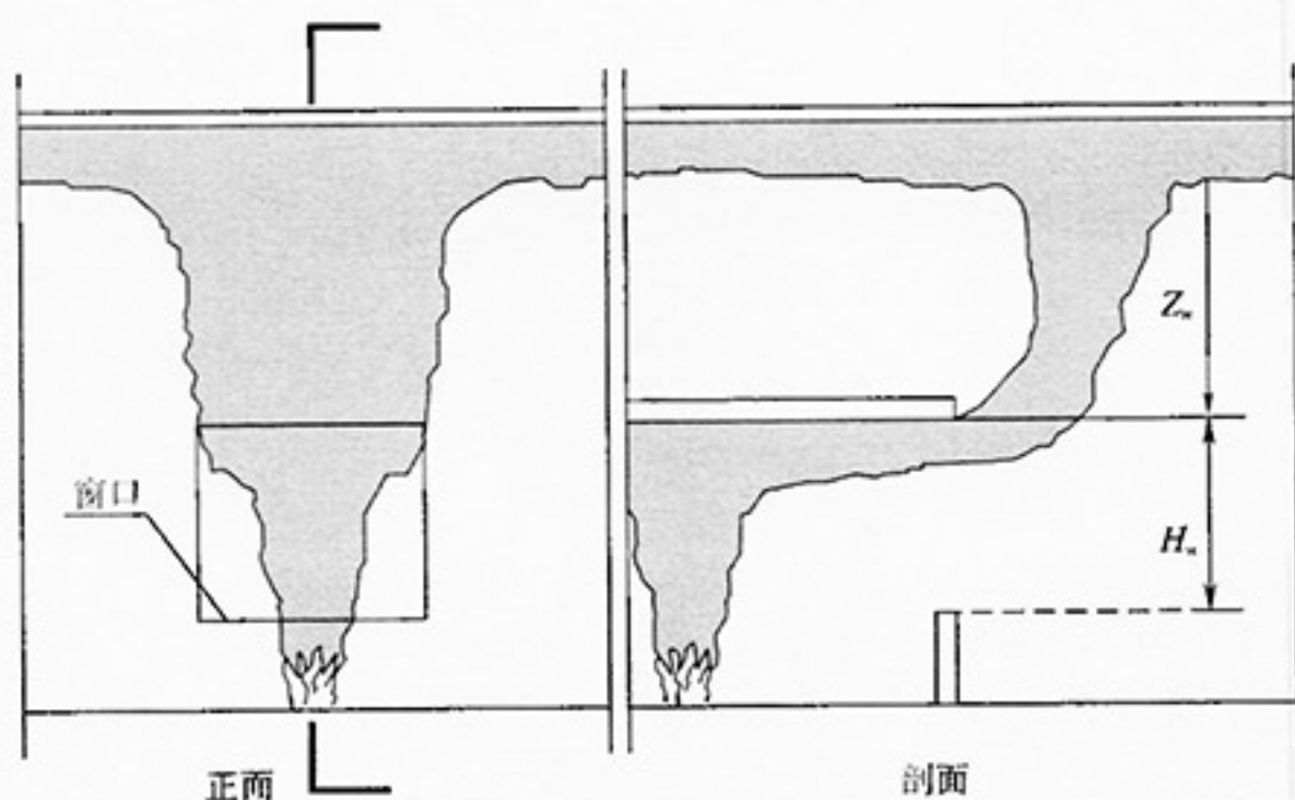
图 12 窗口溢出型烟羽流
