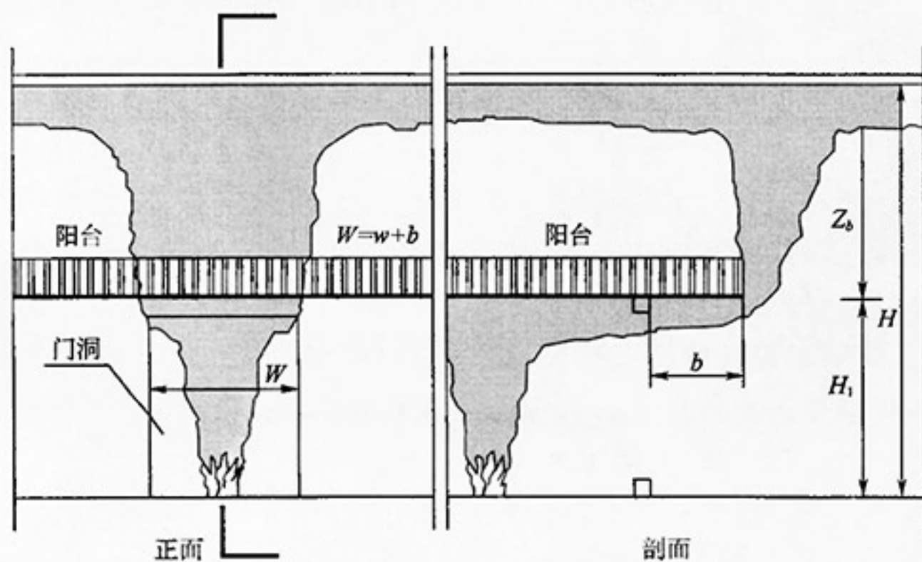
图 11 阳台溢出型烟羽流
