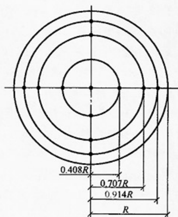
图 18 圆形风管测点布置图
