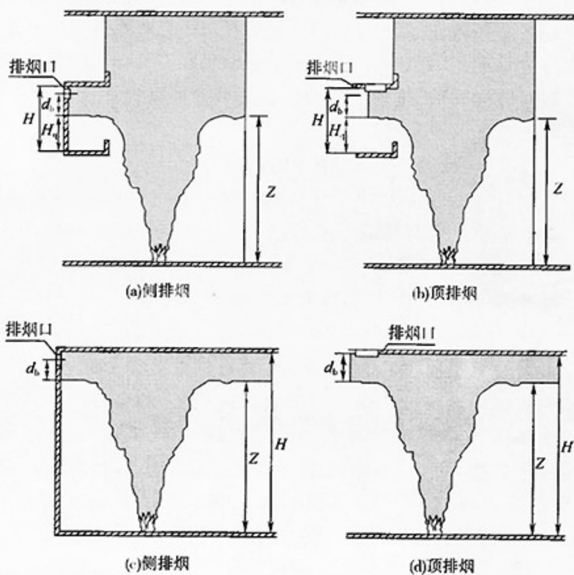
图 16 排烟口设置位置参考图
