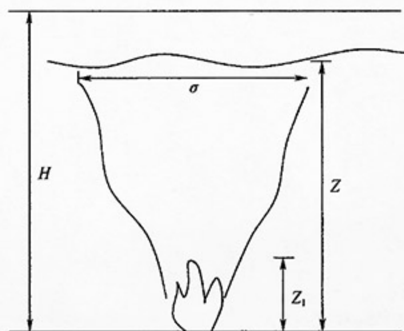
图 10 轴对称型烟羽流
