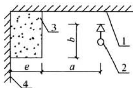
图 7.2.5 喷头与靠墙障碍物的距离
