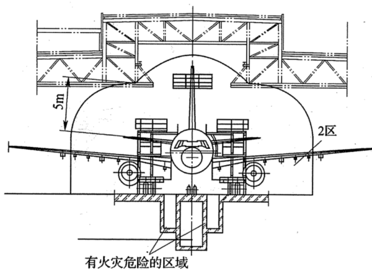
图 3 爆炸危险区域剖面 2
