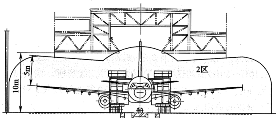
图 2 爆炸危险区域剖面 1
