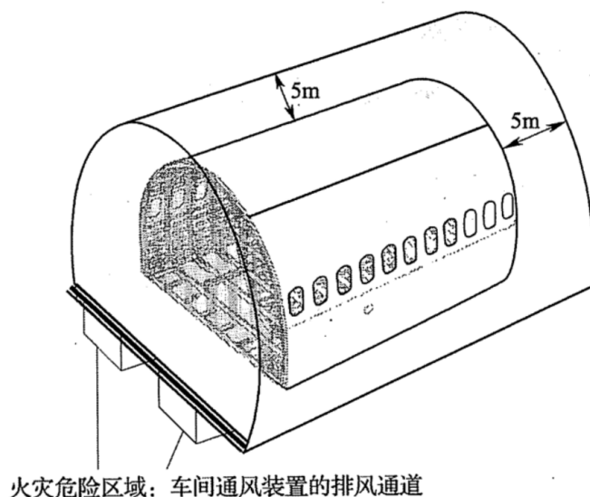
图4 飞机主要部件喷漆爆炸危险区域
