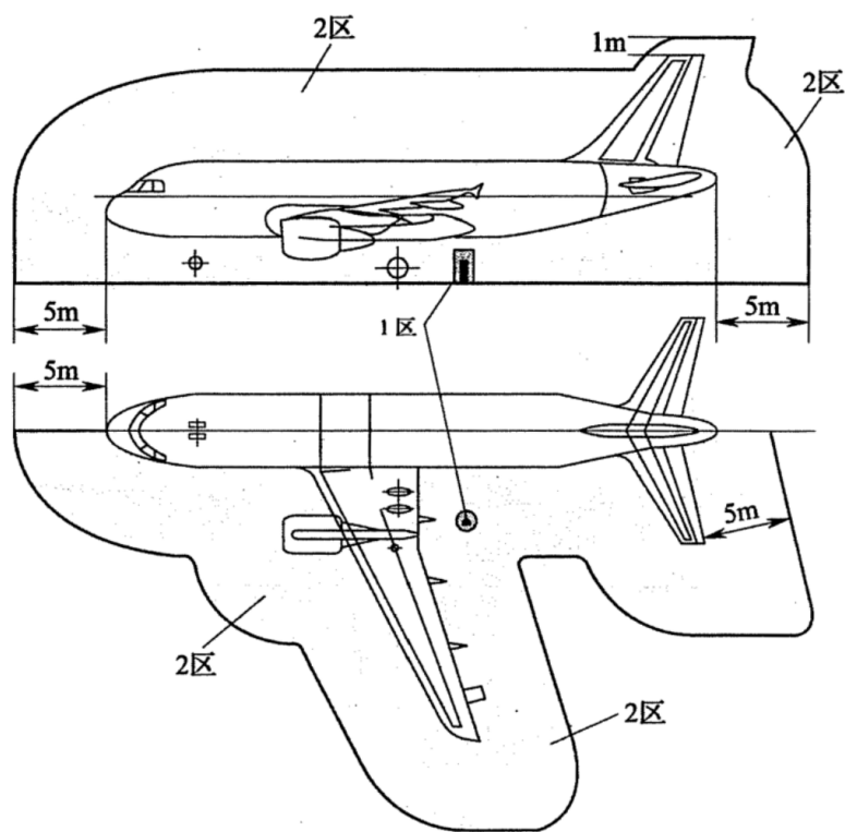
图 1 爆炸危险区域平面
