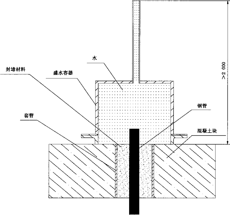
图 C.3 机械管道封堵材料水密试验装置简图
