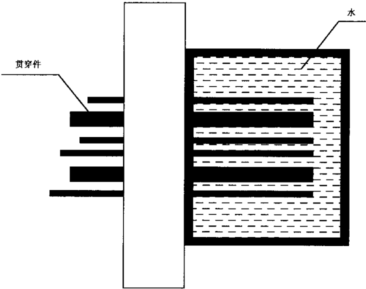
图 C.2 1b 级电缆贯穿防火封堵组件的试验装置
