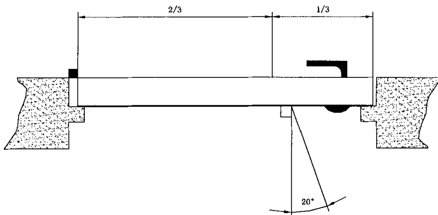
图 D.1 推力作用点位置
