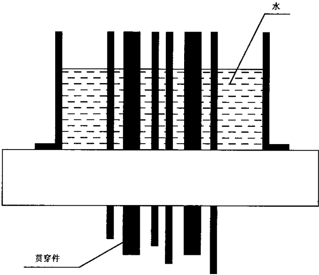
图 C.1 1a 级电缆贯穿防火封堵组件的试验装置
