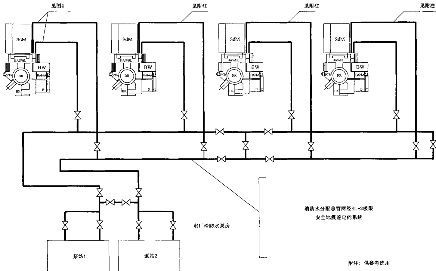
图 1 高压消防水分配原理图
