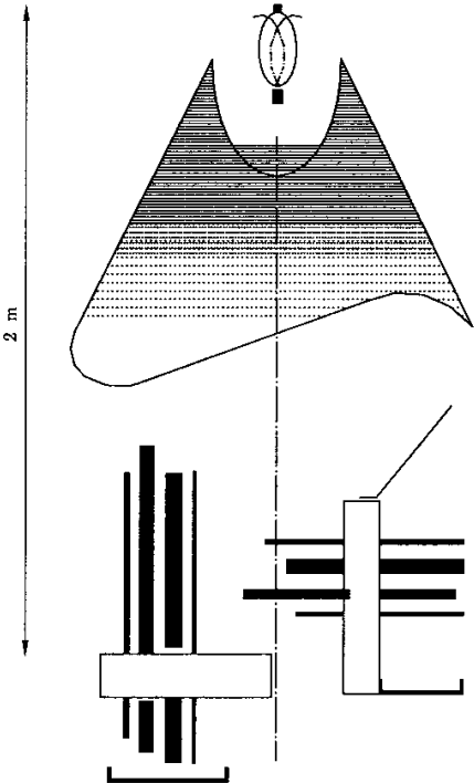
图 C.4 1c 和 1d 级电缆贯穿防火封堵组件的试验装置
